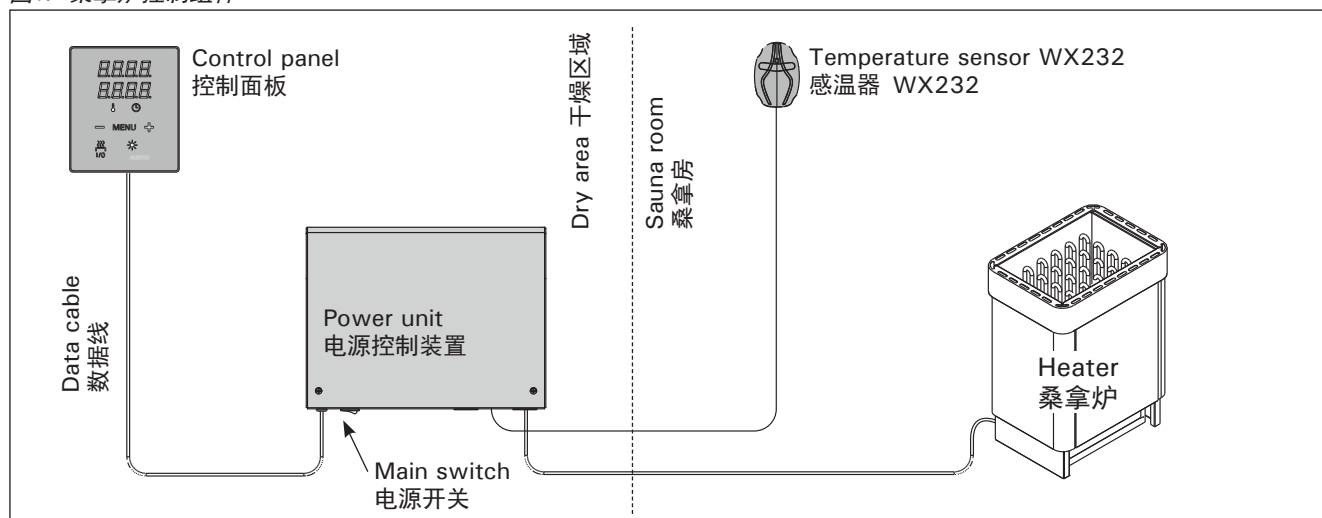
图1. 桑拿炉控制组件
